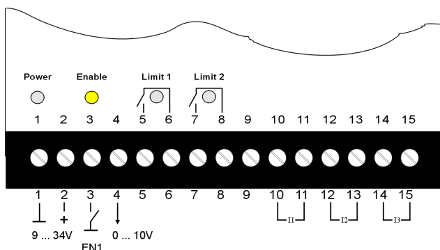
Abbildung 1: Freigabe Eingang Klemme 3 ( für Grenzwertrelais 1 )
