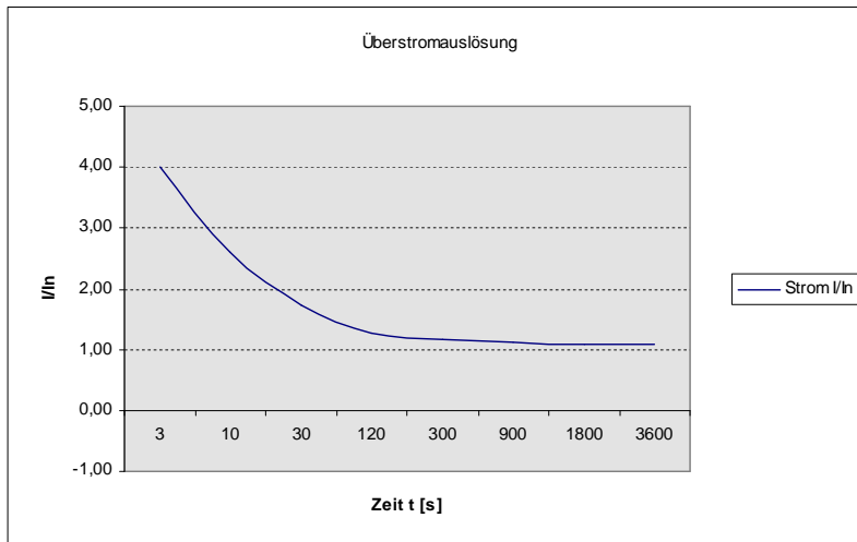
Abbildung 2: stromabhängige Überlastauslösung
